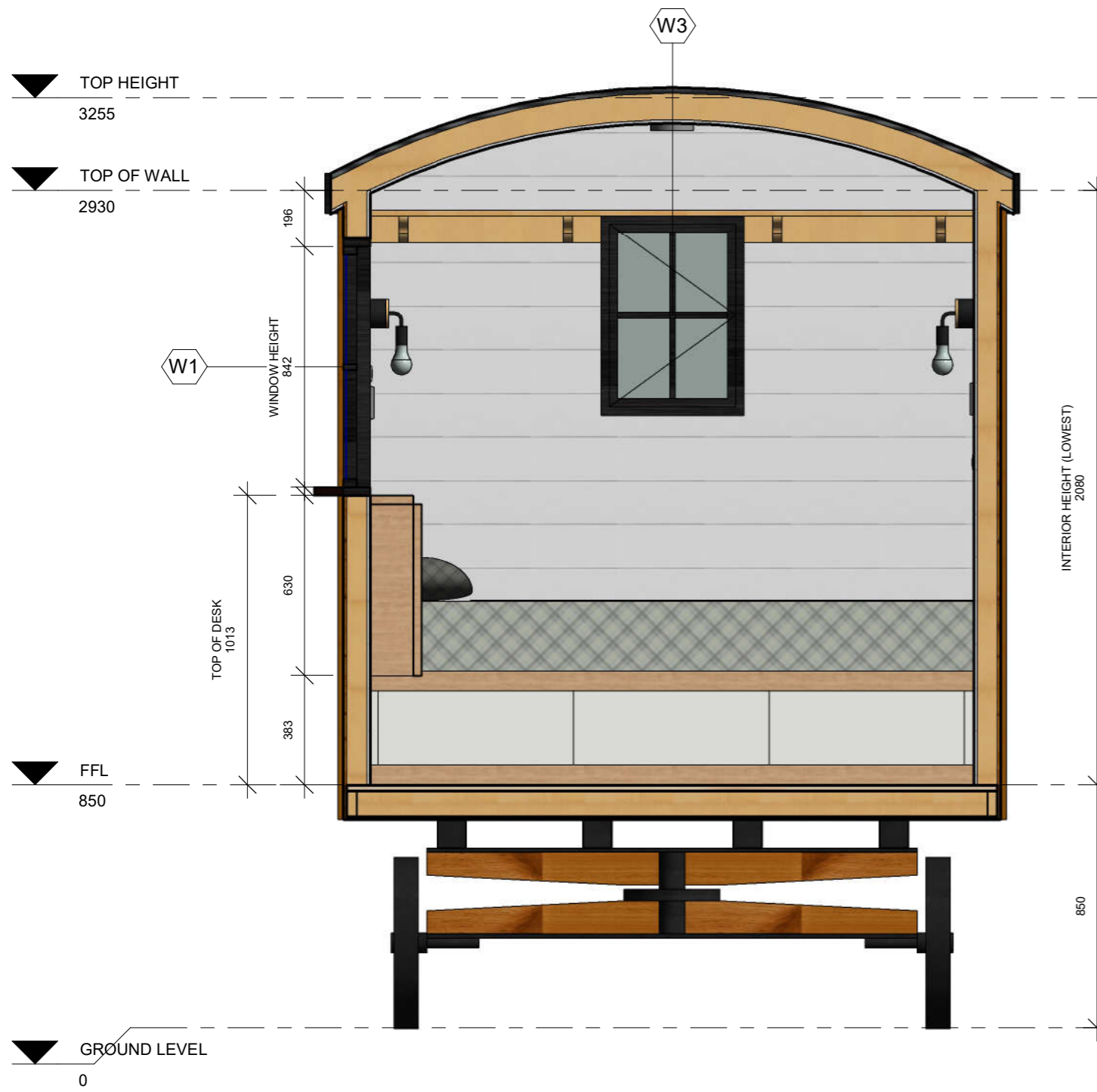
A SECTION A 1 : 20
