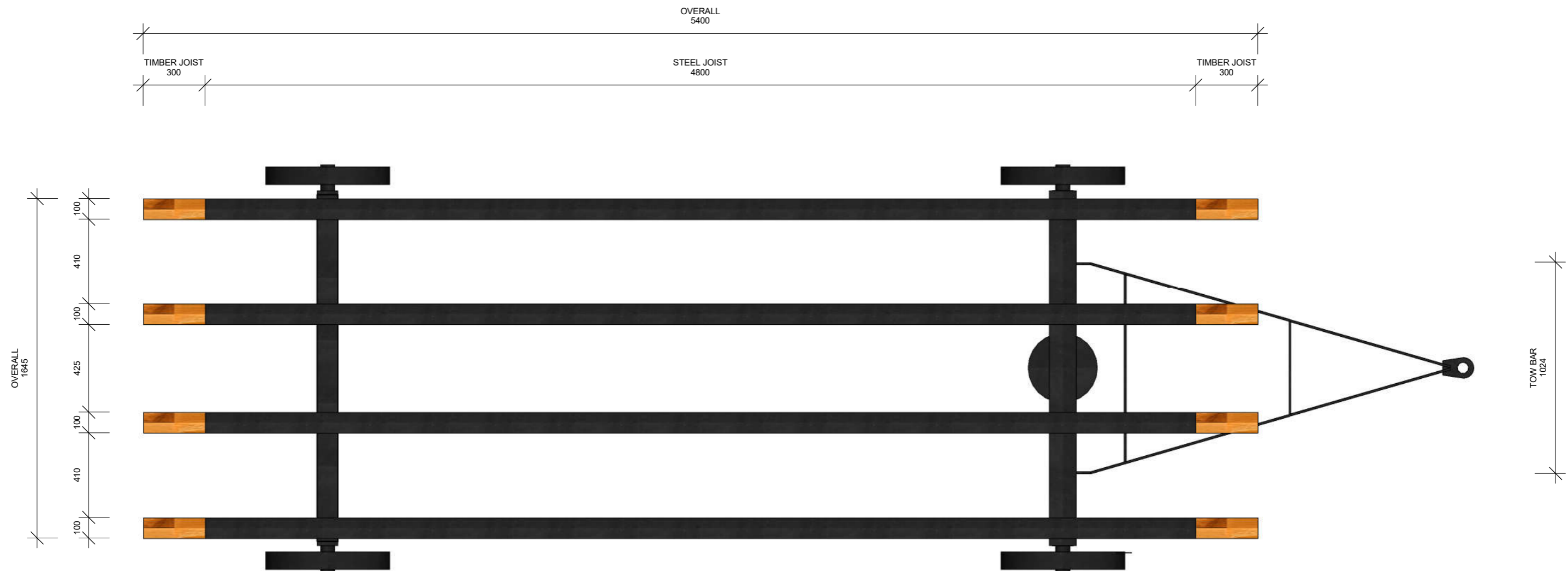
1 TRAILER PLAN 1 : 20
